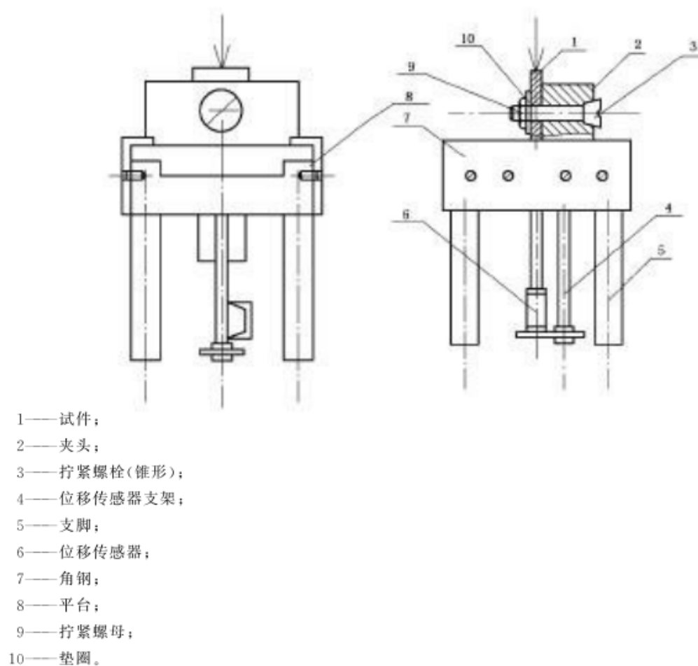
图 4(b) 单搭接压缩型加载装置
